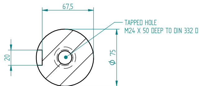
Przekrój A-A 1:2
